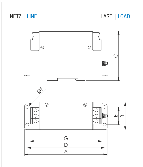
Gehäuse Bauart: NF-BFG-CD, NF-BFG-CD-LL Case style: NF-BFG-CD, NF-BFG-CD-LL
