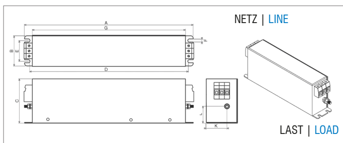
Gehäuse Bauart A: 16 A, 25 A, 40 A | Case style A: 16 A, 25 A, 40 A
