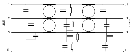
Prinzipschaltbild 3ph-Filter:
