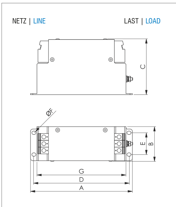
Gehäuse Bauart: NF-BFG, NF-BFG-LL Case style: NF-BFG, NF-BFG-LL
