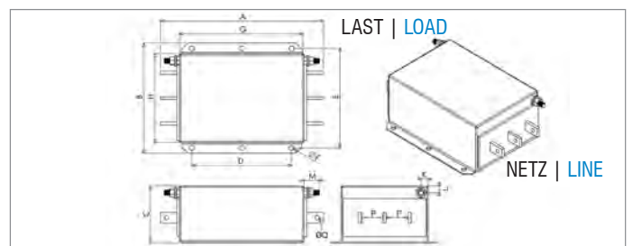
NF-DAR-300-3
