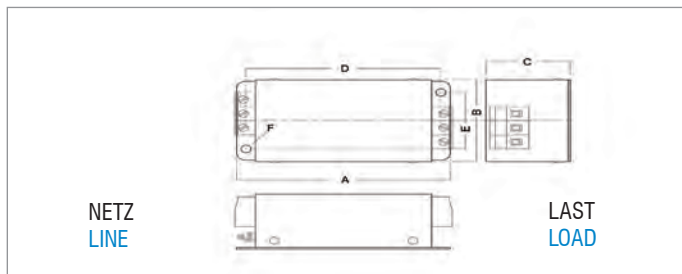
NF-DAR-10-3
