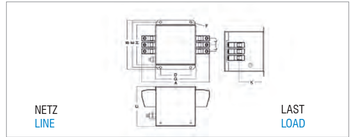
NF-DAR-50-3
