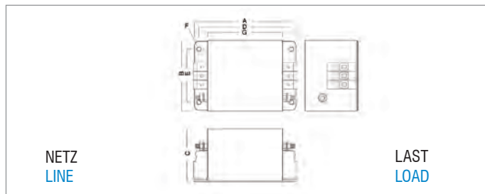
NF-DAR-40-3
