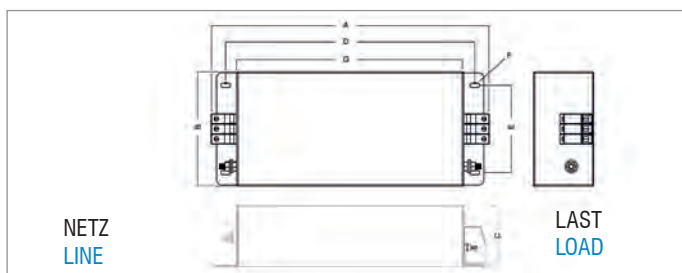
NF-DAR-180-3
