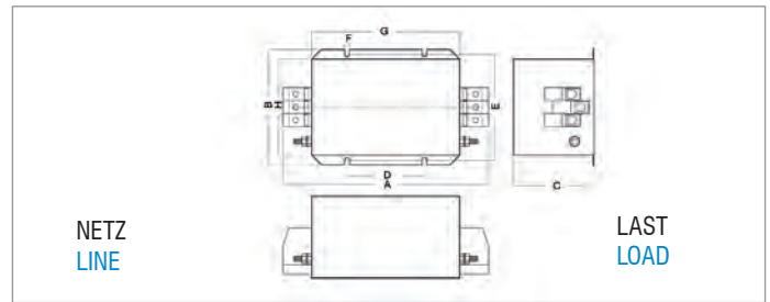
NF-DAR-125-3, NF-DAR-150-3
